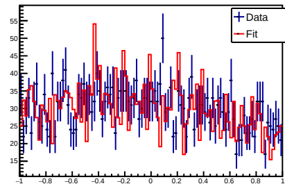
Theta (Lambda_HeliXibarpLambdaKm)
