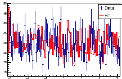
Phi (Lambda_HeliXibarpLambdaKm)
