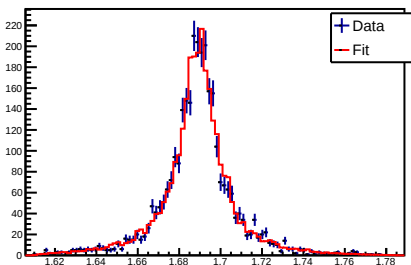
M(LambdaKm)
