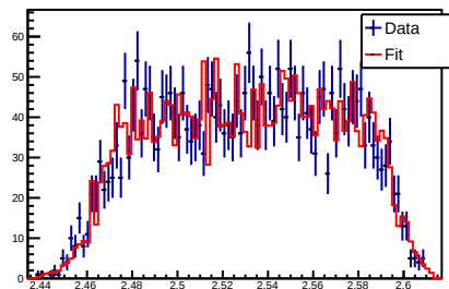
M(XibarpLambda)
