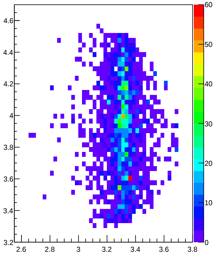
\Xi^+ \Lambda K^- Data
