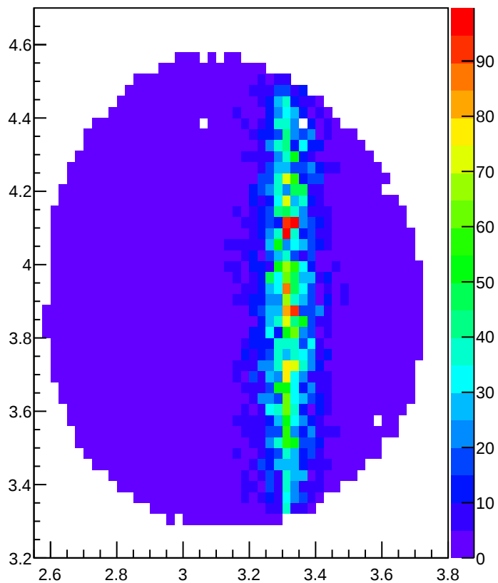
\Xi^+ \Lambda K^- Fit
